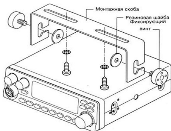
Рис. 1. Крепление радиостанции при помощи монтажной скобы.
