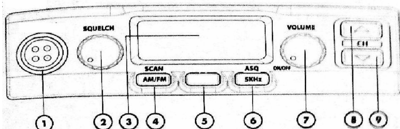
Рис. 1. Органы управления радиостанцией указаны цифрами.
