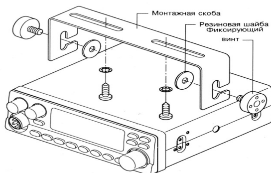
Рис. 1. Крепление радиостанции при помощи монтажной скобы.
