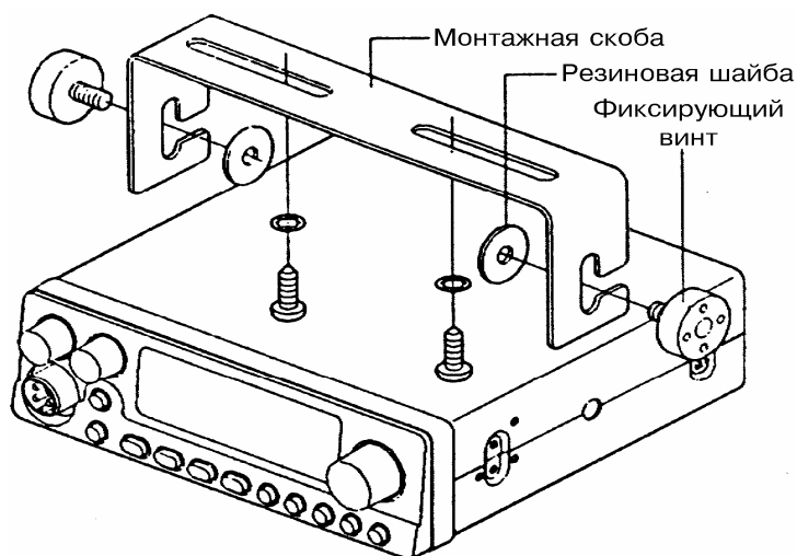
Рис.2. Крепление радиостанции при помощи монтажной скобы.
