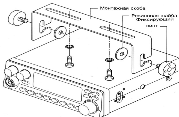
Рис.1. Крепление радиостанции при помощи монтажной скобы.
