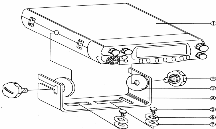
Рис. 4. Крепление радиостанции при помощи монтажной скобы.
